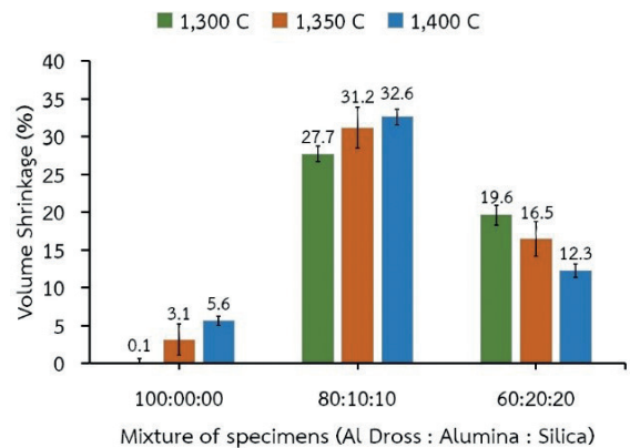
รูปที่ 9 ร้อยละการหดตัวเชิงปริมาตรของตะกรัน อะลูมิเนียม : อะลูมินา : ซิลิกา ที่ 100 : 0 : 0, 80 : 10 : 10 และ 60 : 20 : 20 อุณหภูมิเผาประสาน 1,300 1,350 และ 1,400 องศาเซลเซียส
