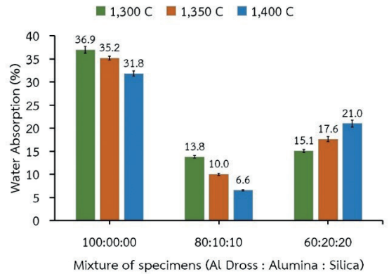
รูปที่ 15 ร้อยละการดูดซึมน้ำของตะกรันอะลูมิเนียม : อะลูมินา : ซิลิกา ที่ 100 : 0 : 0, 80 : 10 : 10 และ 60 : 20 : 20 อุณหภูมิเผาประสาน 1,300 1,350 และ 1,400 องศาเซลเซียส
