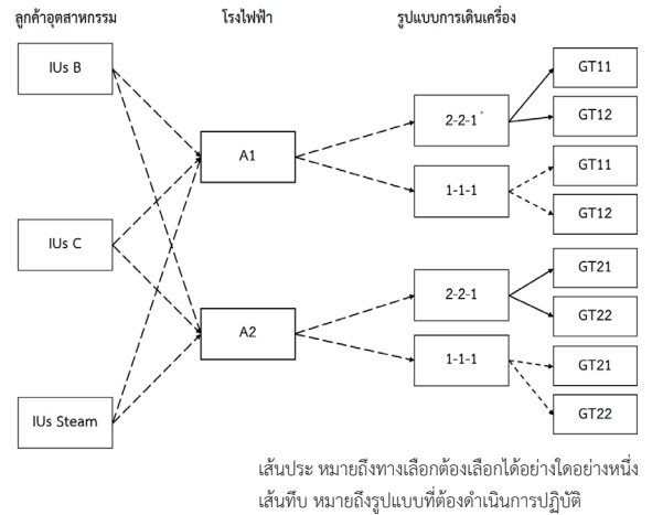
รูปที่ 1 รูปแบบการเดินเครื่องของบริษัท AAA จำกัด
