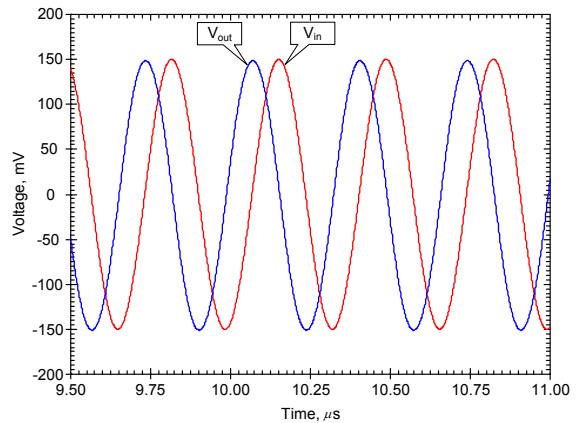
รูปที่ 6 รูปคลื่นอินพุตและเอาต์พุตเมื่อป้อนอินพุตความถี่ 2.98 MHz ขนาด 300\text{mV}_{p-p}
