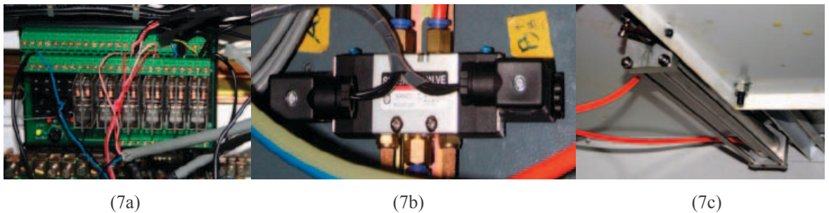
รูปที่ 7 ระบบเปิด-ปิดประตูอัตโนมัติของเครื่องกัดซีเอ็นซี (7a) การต่อสายสัญญาณเข้าวงจรรีเลย์ (7b) การต่อสายสัญญาณเข้าโซลินอยด์วาล์ว (7c) การติดตั้งกระบอกลมเพื่อเปิด-ปิดประตู
