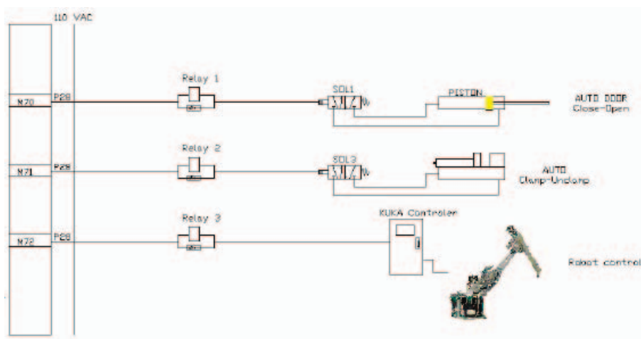
รูปที่ 5 รูปแบบวงจรการนำเอาท์พุตจาก I/O Board ไปใช้งาน
