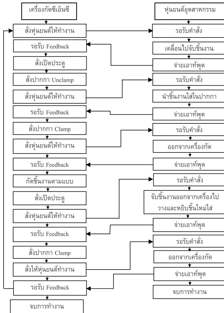
รูปที่ 2 ความสัมพันธ์ของลำดับการทำงานระหว่างเครื่องกัចซีเอ็นซีและหุ่นยนต์อุตสาหกรรม
