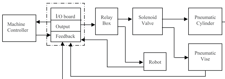
รูปที่ 2 ความสัมพันธ์ของลำดับการทำงานระหว่างเครื่องกัចซีเอ็นซีและหุ่นยนต์อุตสาหกรรม
