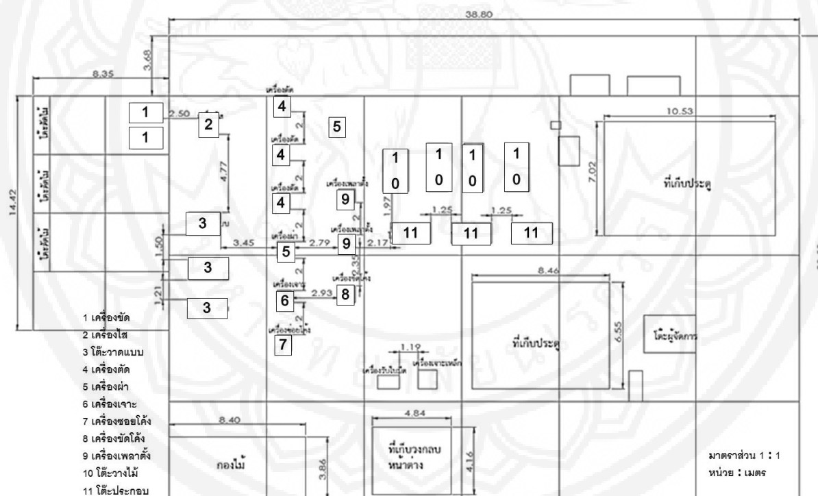
รูปที่ 7 ผังโรงงานหลังการปรับปรุง
