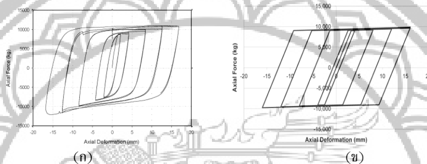
รูปที่ 5 พฤติกรรมภายใต้แรงวัฏจักร (Hysteretic behavior) (ก) จากผลการทดสอบ (ข) จากแบบจำลอง
