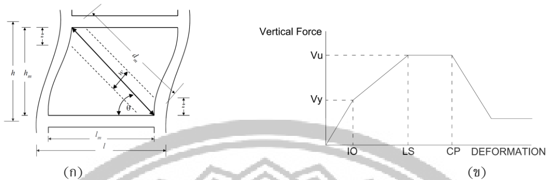
รูปที่ 3 (ก) พฤติกรรมของผนังอิฐก่อภายใต้แรงกระทำทางด้านข้าง
