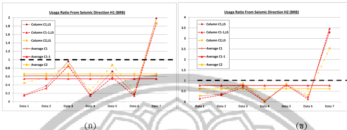
รูปที่ 11 ค่า Demand-Capacity Ratio(DCR)การวิเคราะห์ตามประวัติเวลาแบบไม่เชิงเส้นด้วยคลื่นแผ่นดินไหวหลังเสริมกำลังด้วย BRB (ก) สำหรับทิศทางตามขวาง (ข) สำหรับทิศทางตามยาว
