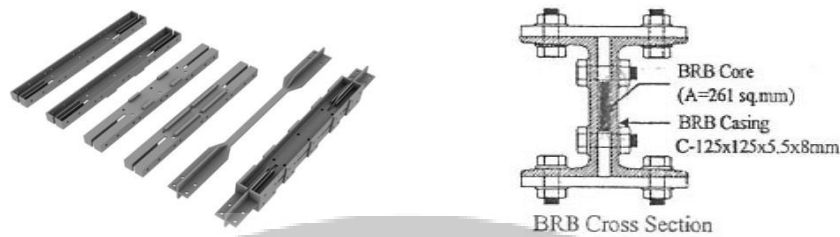
รูปที่ 4 รูปแบบขององค์อาคารยึดไร้การโก่งเดาะ
