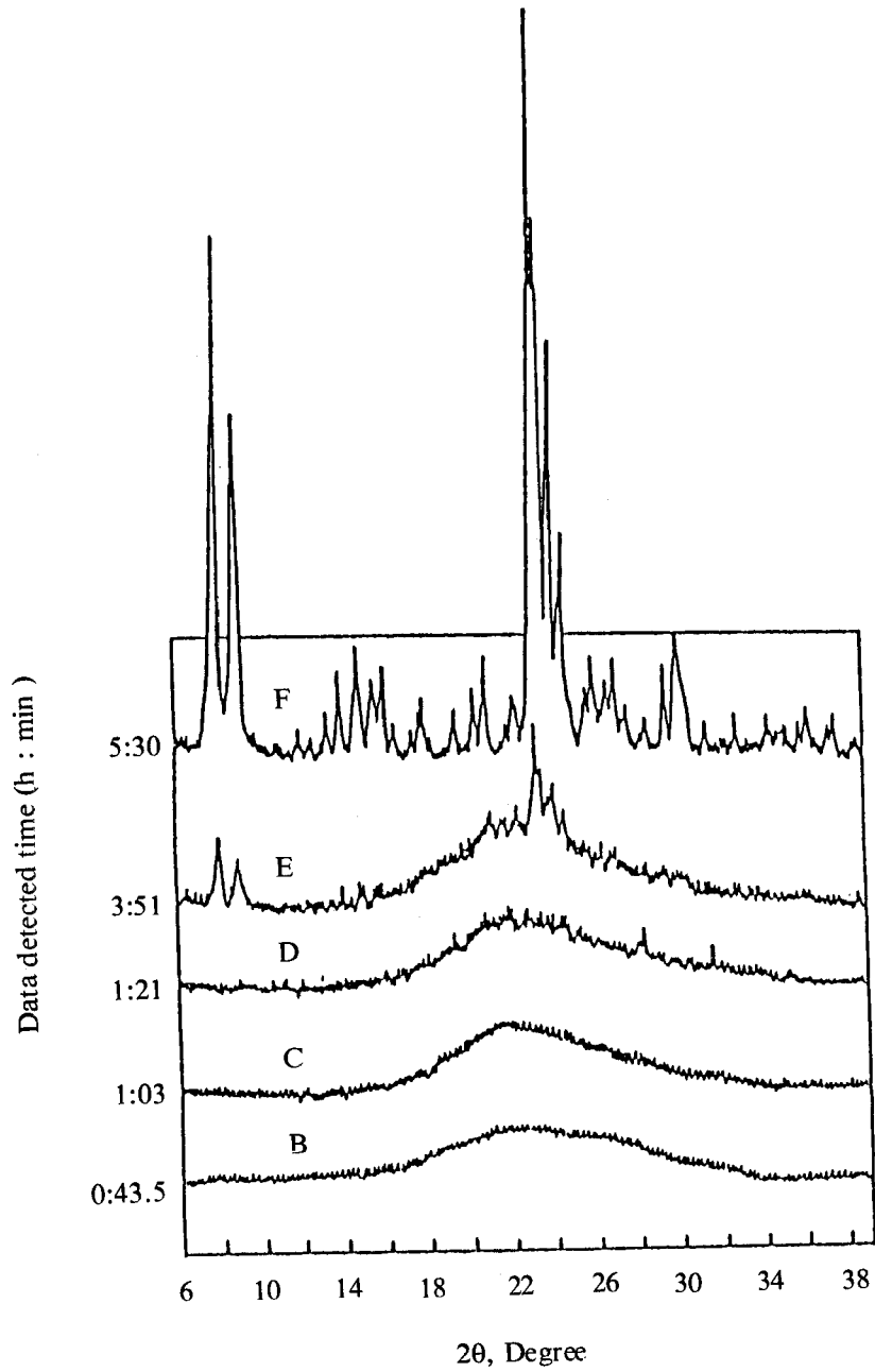
รูปที่ ๑. รูปแบบ XRD ของผลิตภัณฑ์ผลึกที่เกิดขึ้นในช่วงระยะเวลาต่างๆ ตามจุดที่กำหนด
