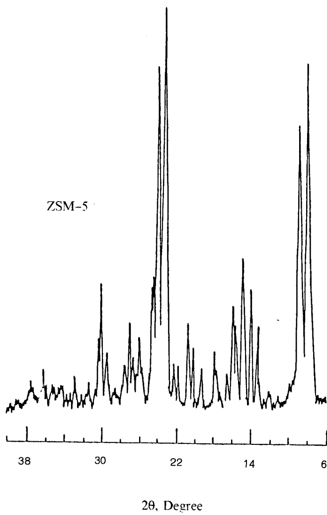
รูปที่ 6. รูปแบบมาตรฐาน XRD ของ ZSM-5 zeolite 3
