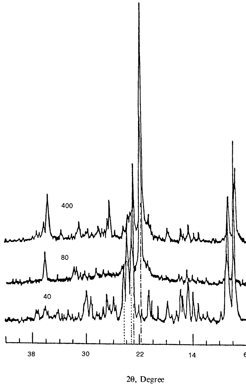
รูปที่ 5. รูปแบบ XRD ของผลิตภัณฑ์ผลึกที่อัตราการเพิ่มอุณหภูมิอัตราที่ II สำหรับ Si/Al = 40, 80 และ 400 ตามลำดับ
