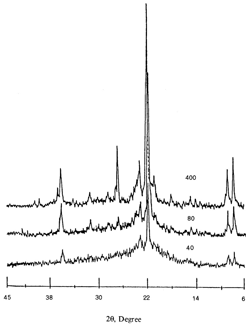
รูปที่ 4. รูปแบบ XRD ของผลิตภัณฑ์ผลึกที่อัตราการเพิ่มอุณหภูมิอัตราที่ I สำหรับ Si/Al = 40, 80 และ 400 ตามลำดับ
