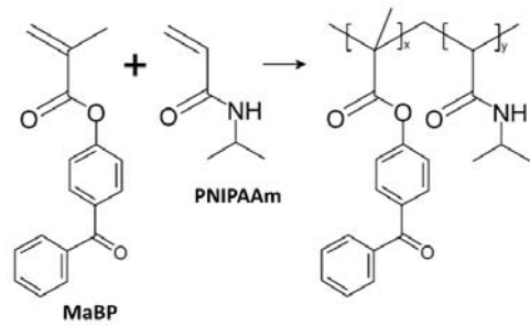
รูปที่ 5 การเตรียมโคพอลิเมอร์ของ PNIPAAm/MaBP [7]
