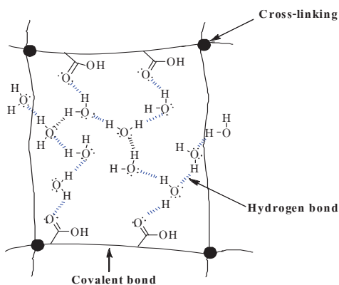
รูปที่ 1 กลไกการดูดน้ำของ poly(sodium acrylate) [3]
