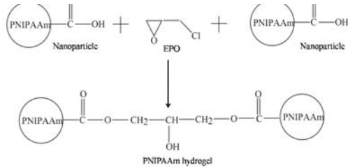
รูปที่ 3 แผนภาพการเตรียม PNIPAAm hydrogel [5]
