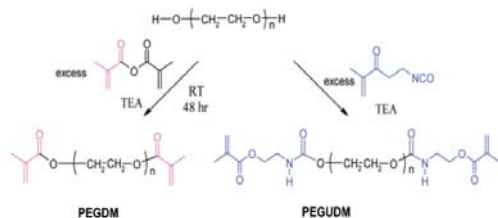
รูปที่ 18 การสังเคราะห์ไฮโดรเจลชนิด PEGDM และ PEGUDM [24]
