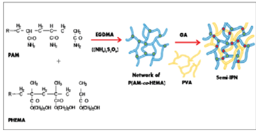
รูปที่ 7 การเตรียม P(AM-co-HEMA)/PVA semi-IPN hydrogel [9]
