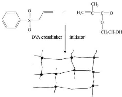
รูปที่ 13 การสังเคราะห์ไฮโดรเจลชนิด APS-co-HEMA hydrogels [15]
