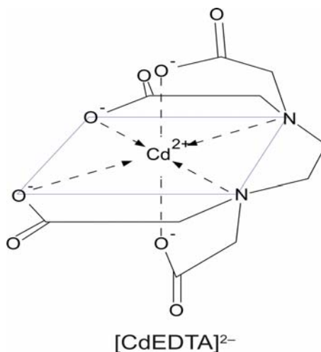
รูปที่ 41 การเกิดสารประกอบเชิงซ้อนระหว่าง EDTA กับโลหะหนัก [50]
