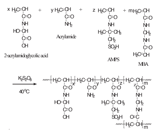
รูปที่ 6 สมการแสดงปฏิกิริยาการสังเคราะห์ AAm/AAGA/AMPS ไฮโดรเจล [8]
